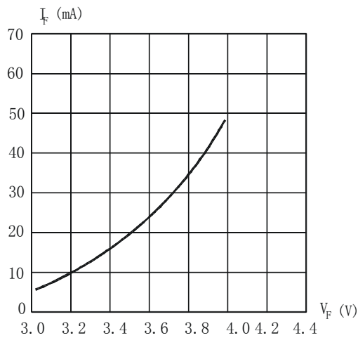
正向电流与正向电压曲线图
