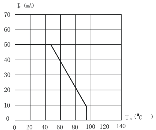
最大正向直流电与温度曲线图
