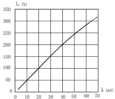
光强与正向电流曲线图
