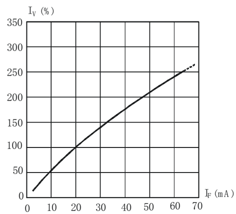
光强与正向电流曲线图
