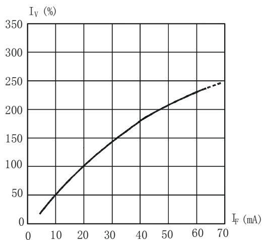
光强与正向电流曲线图
