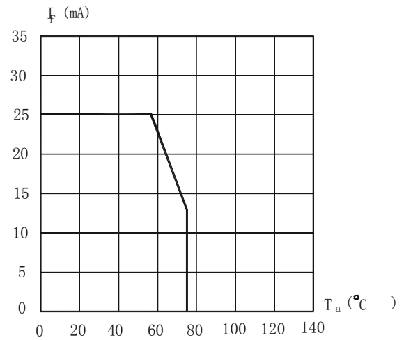
最大正向直流电与温度曲线图
