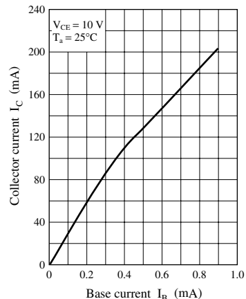
I_C - I_B
