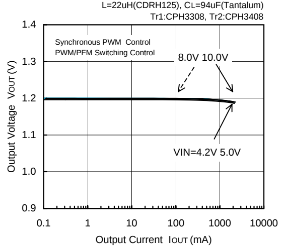
FOSC=300kHz, V_{OUT}=1.2V
