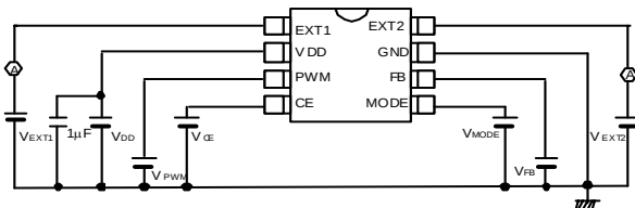
Circuit 1 :
