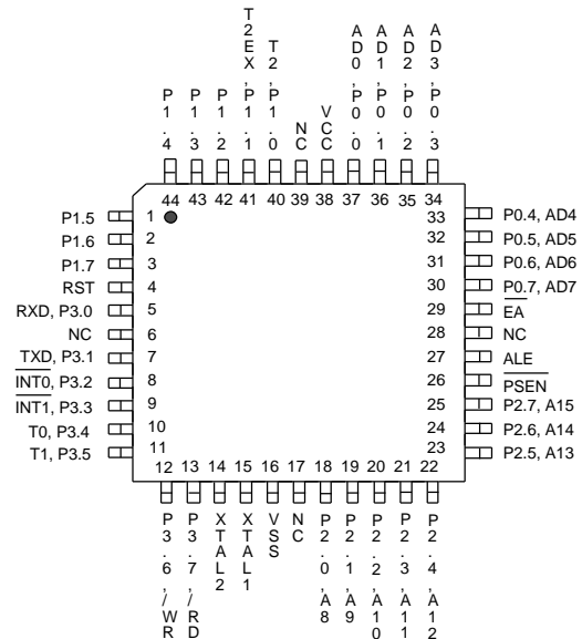
44-Pin QFP/TQFP (W78C52CF/W78C52CM)
