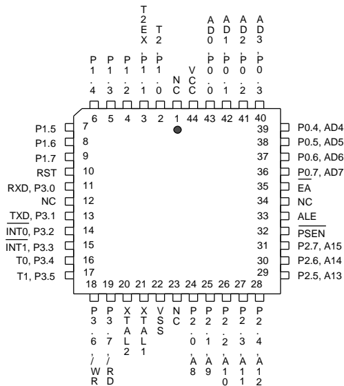
44-Pin PLCC (W78C52CP)
