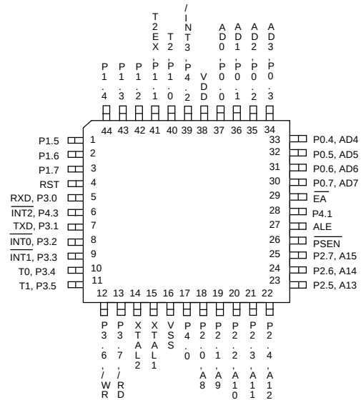
44-Pin QFP (W78E58BF)
