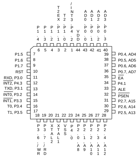
44-Pin PLCC (W78E58BP)
