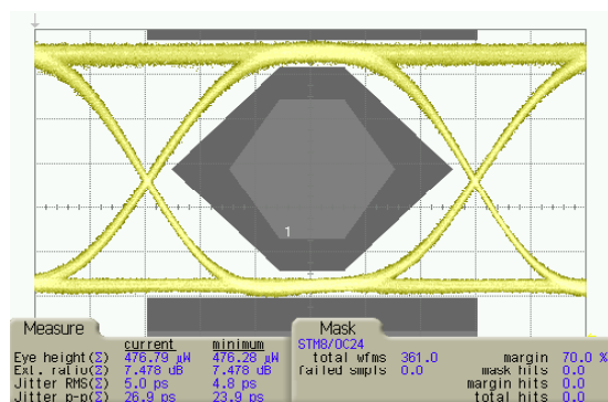
1.25Gbps eye diagram
