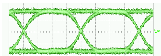
2.5Gbps eye diagram
