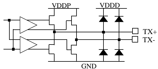
Hi Speed Outputs (TX+/-)
