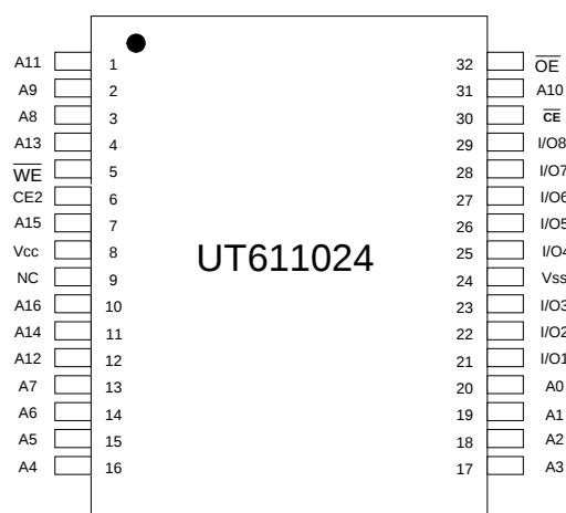
STSOP / TSOP-1
