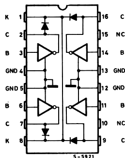
ULN2064B ULN2066B
