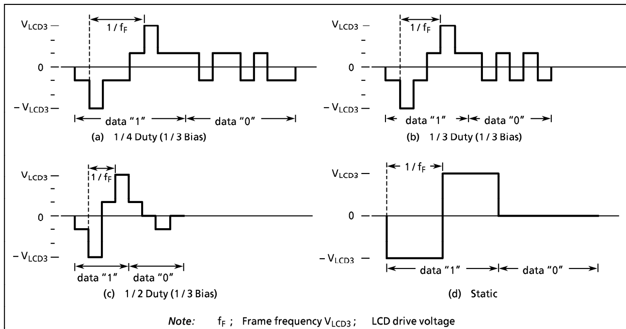
Figure 2-45. LCD Drive Waveform (COM – SEG pins)
