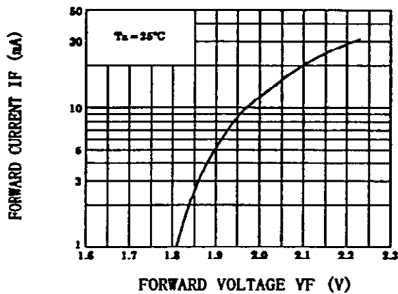
IF - VF
