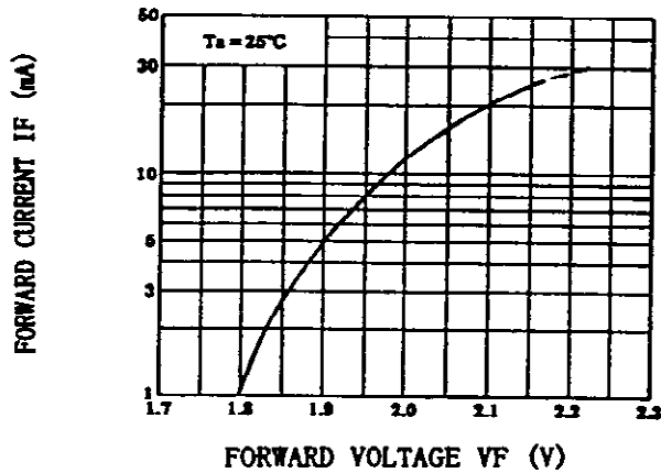
IF - VF
