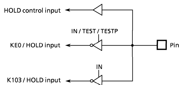
Figure 3-9. Port KE
