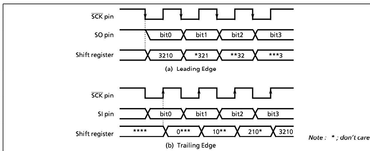
Figure 2-35. Shift Edge
