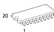
F (SOP20—P—300) Weight : 0.22g (TYP.)
