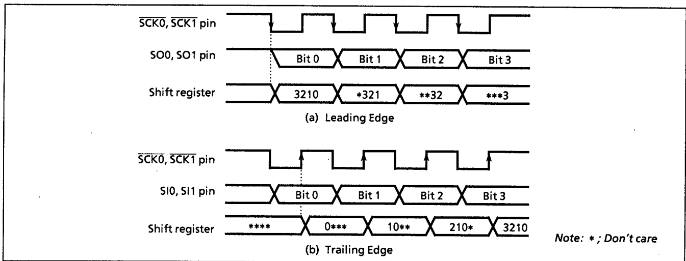
Figure 2-53. Shift Edge
