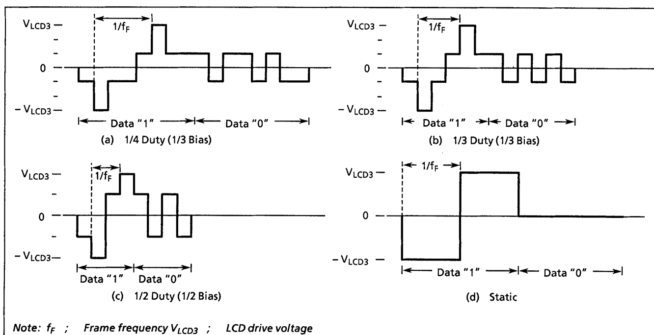
Figure 2-68. LCD Drive Waveform (COM - SEG pins)
