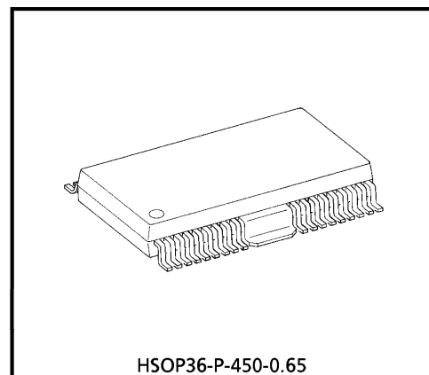
HSOP36-P-450-0.65 Weight : 0.79 g (Typ.)
