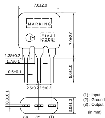
SFELA10M7GALP03-B0
