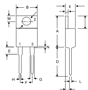
TO-220A
