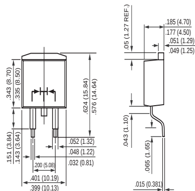
D2PAK
