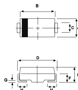
DO-214AC(SMA)
