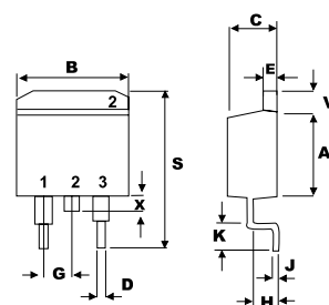
TO-263 (D2-PAK)
