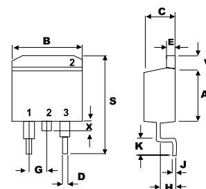
TO-263 (D2-PAK)
