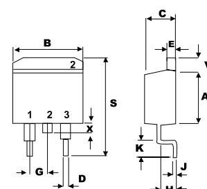
TO-263 (D2-PAK)
