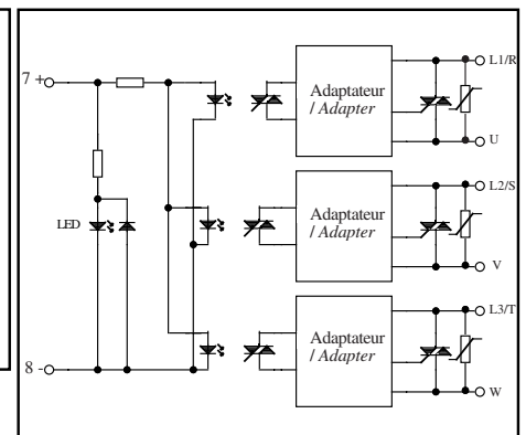
Circuit équivalent/Equivalent circuit :
