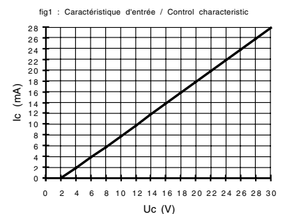
fig. 1 :Caractéristique d'entrée / Control characteristic PER INPUT
