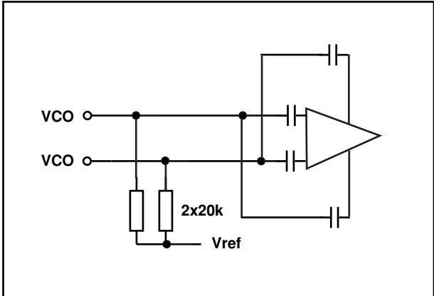
VCO
