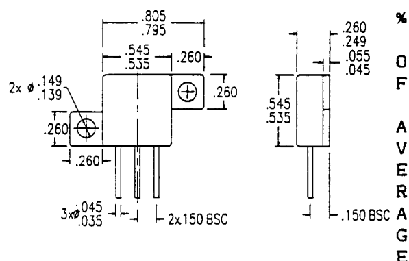
T0-254(M)
