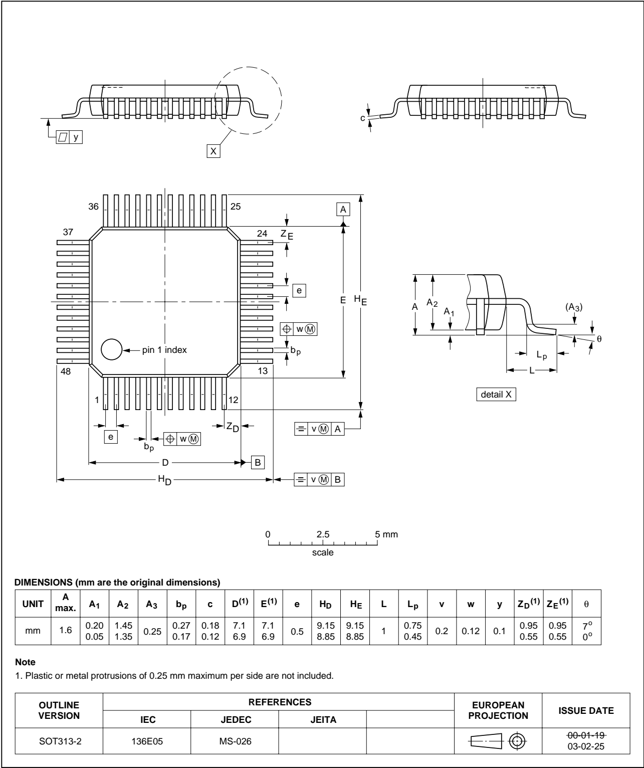
Fig 24. LQFP48 (SOT313-2).
