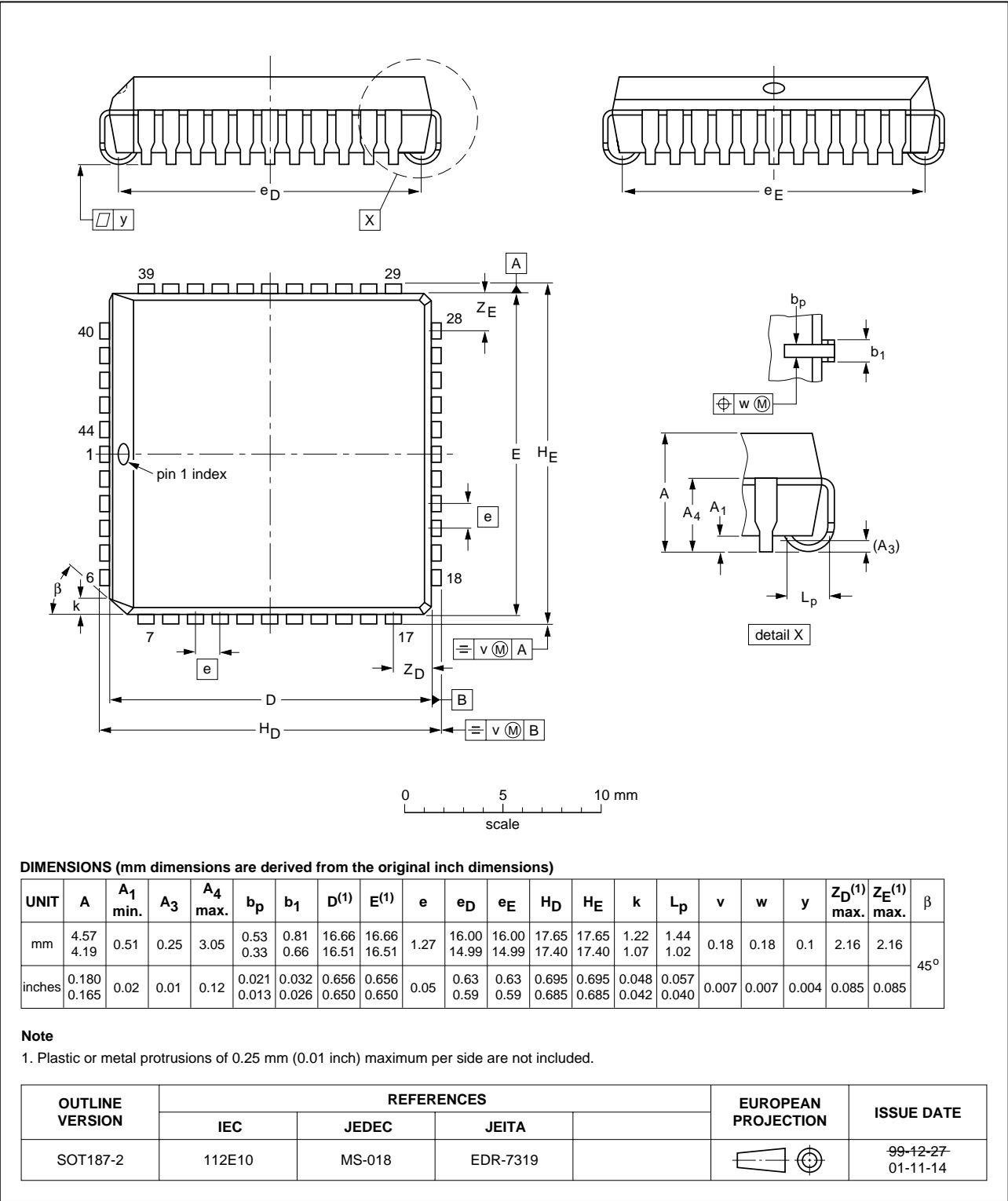
Fig 23. PLCC44 (SOT187-2).
