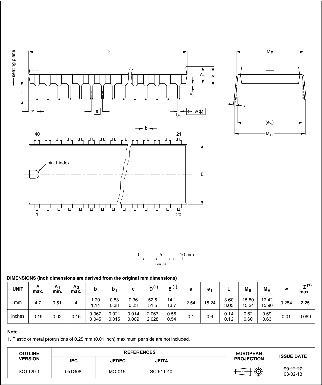
Fig 25. DIP40 (SOT129-1).
