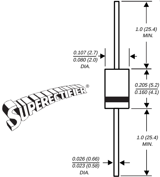
Case Style GP10E
