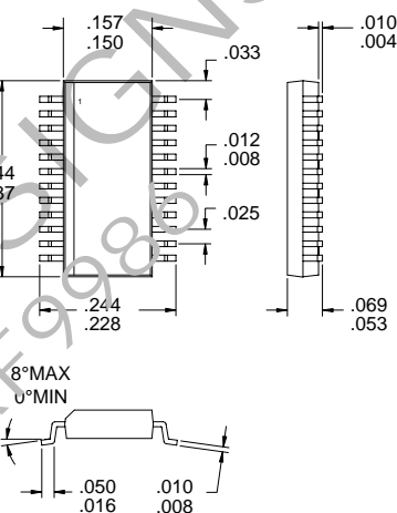
Package Style: SSOP-24
