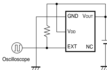
Test Circuit4
