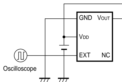
Test Circuit2
