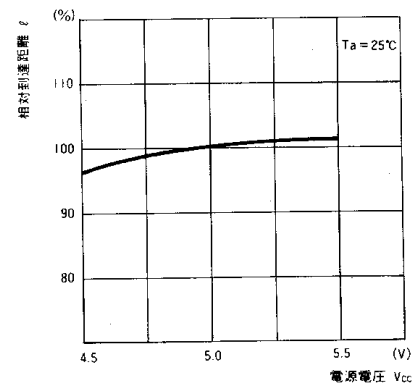
■到達距離/電源電圧特性 \ell/V_{CC}
