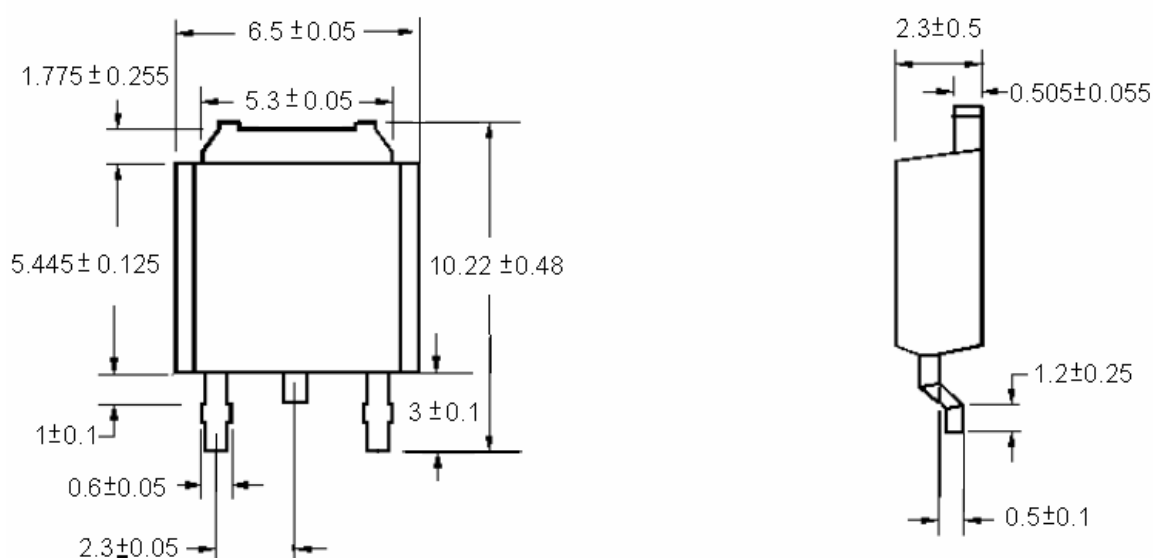
TO-252 Unit:mm
