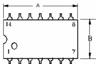
DIP-14
