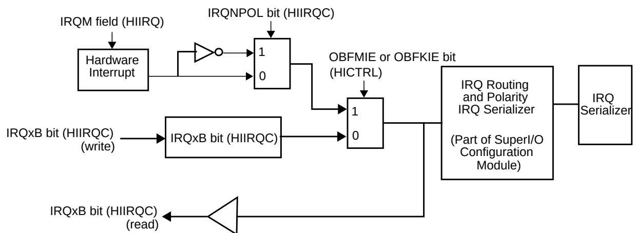
Figure 91. IRQx (IRQ1, IRQ11 or IRQ12) Control Diagram
