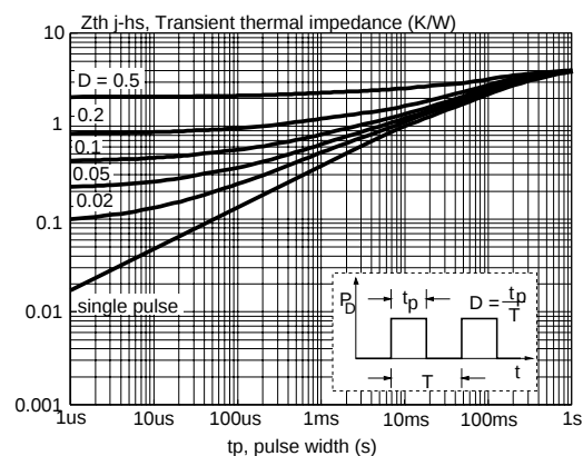
Fig.4. Transient thermal impedance. Z_{th\ j\text{-}hs} = f(t) ; parameter D = t_p / T
