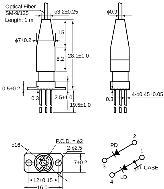
NDL7705P2
