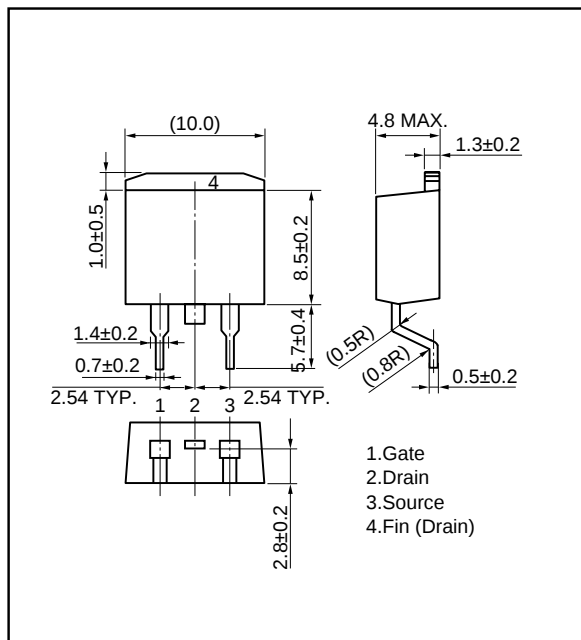
3) TO-263 (MP-25J)
