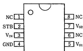
NJU7204XM
