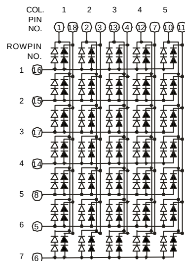
LMD30058B
