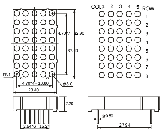
LMD14058A
