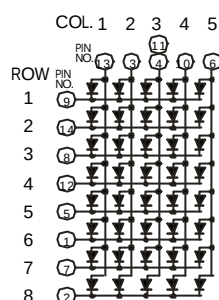
LMD14058A
