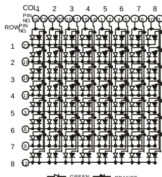
LMD12088A
