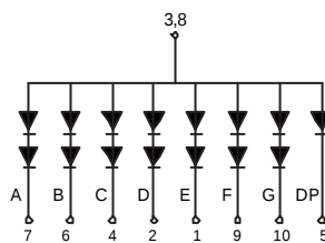
LSD102B
