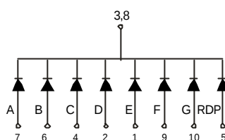
LSD080A
