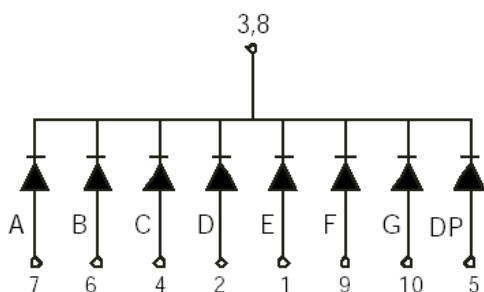
LSD055AG-10
