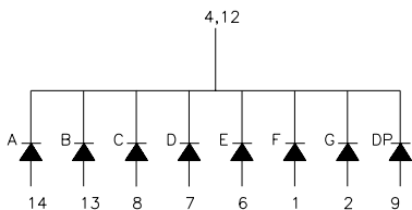
D.LTS-4X40A
